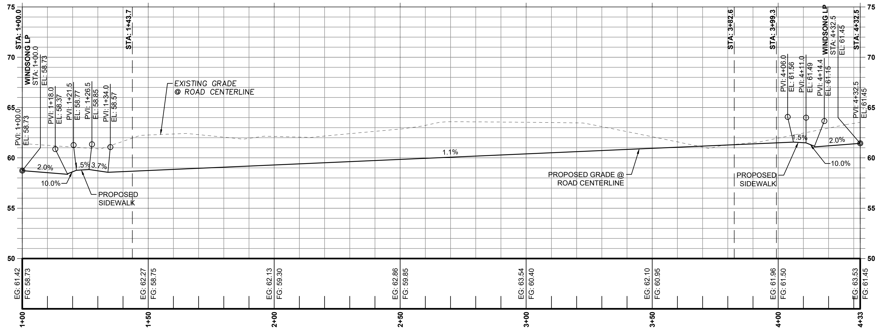
AUTUMN GOLD LN PROFILE (STA: 1+00 - STA: 4+33) SCALE: 1" = 20' H; 1" = 5' V
