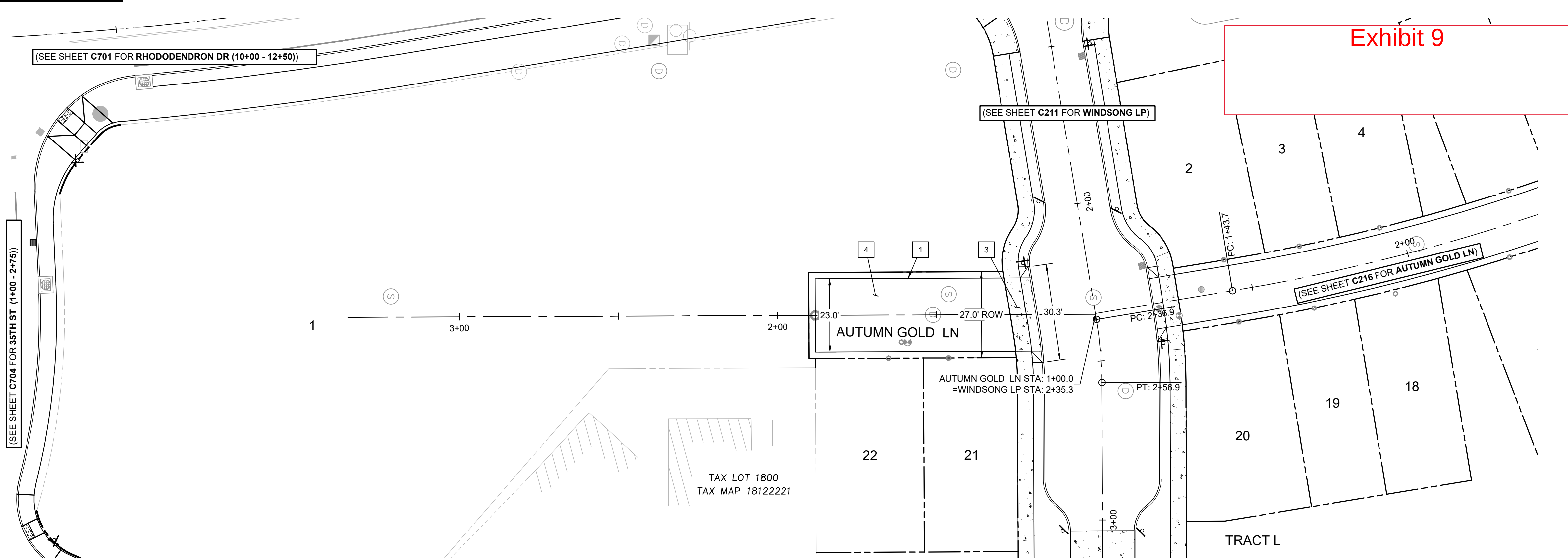
AUTUMN GOLD LN PLAN (STA: 1+00 - STA: 2+25)
