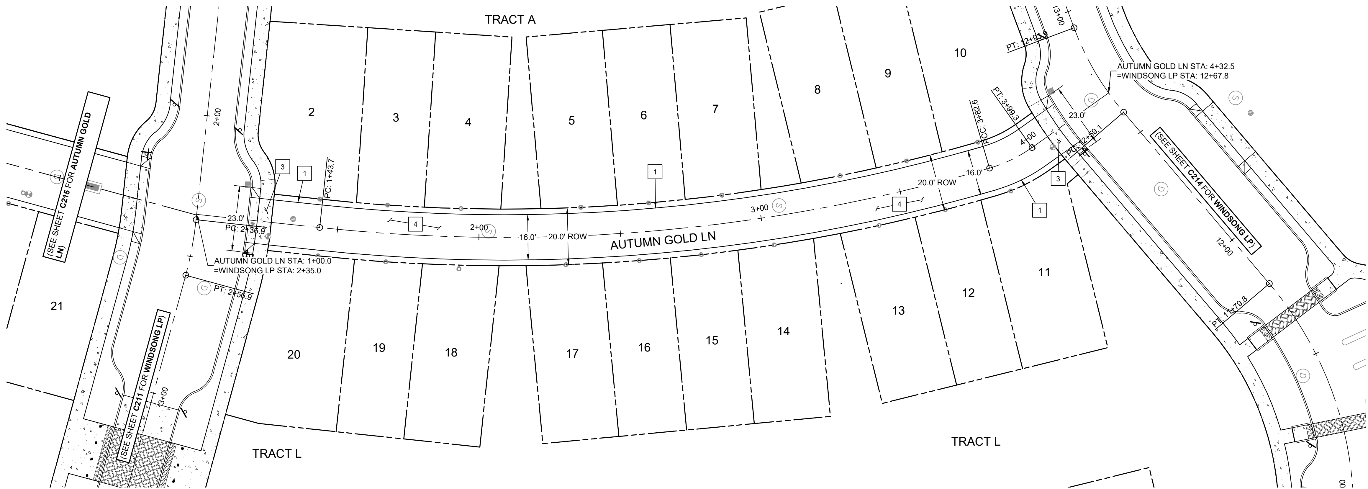
AUTUMN GOLD LANE PLAN (STA: 1+00 - STA: 4+33)
