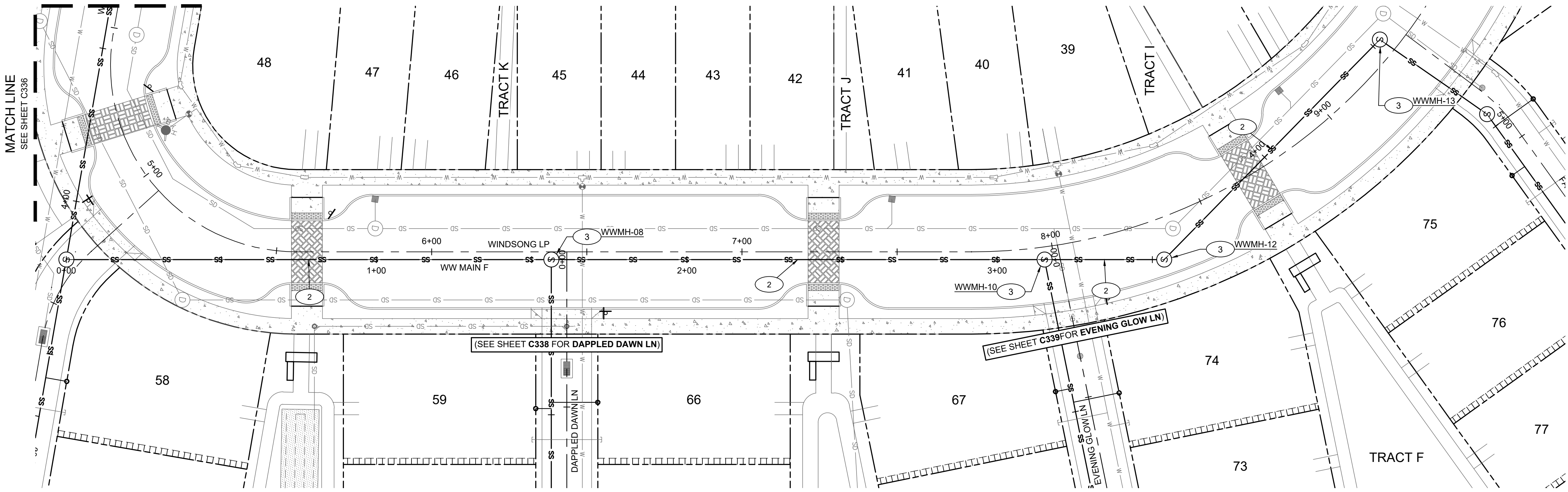
WW MAIN F PLAN (STA: 0+00 - STA: 4+53)
