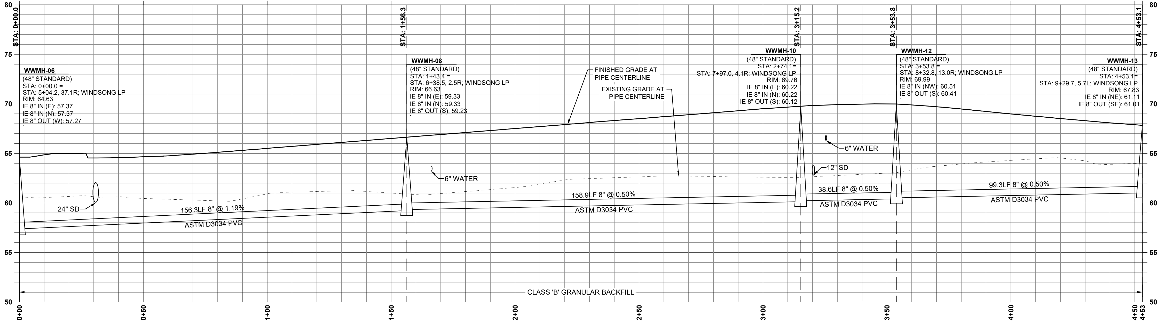
WW MAIN F PROFILE (STA: 0+00 - STA: 4+53) SCALE: 1" = 20' H; 1" = 5' V
